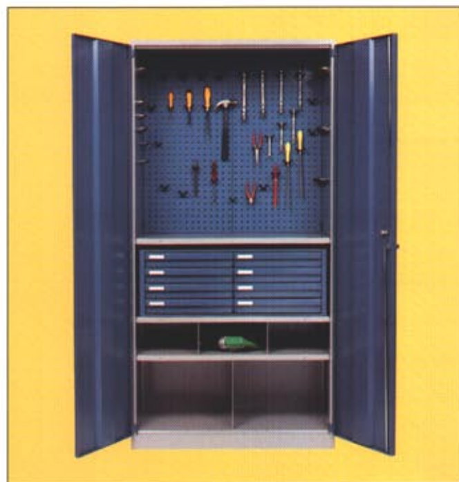
LOCK20 C Består af: 1 skab uden tilbehør 4 hylder (inkl. bundhylde) 2 skilleplader i højde 200 mm 1 skilleplade i højde 400 mm 1 skuffesektion med 8 skuffer (tilbehør til skuffer som LOCK20 B) Værktøjspanel i sider og ryg + et komplet sæt ophængskroge
